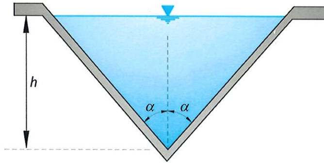
Figura 6.8 Vertedor triangular.
