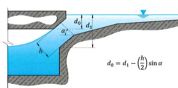
b. Garganta Inclinada
