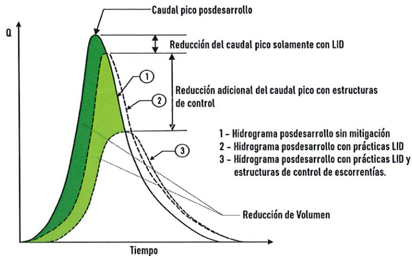
Figura 10.2 Hidrogramas conceptuales de caudales mostrando el concepto de la reducción del caudal pico y volumen de escorrentía postdesarrollo.
