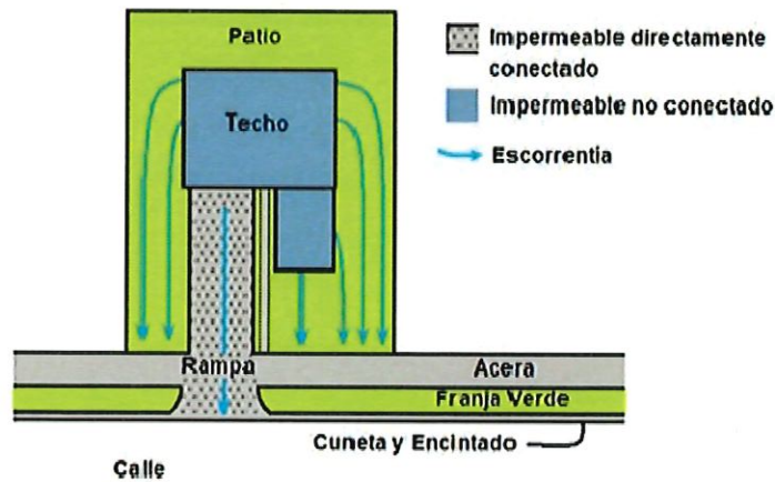
Figura 3.2 Escorrentía de áreas de captación compuestas con zonas impermeables directamente conectadas al sistema de drenaje pluvial
