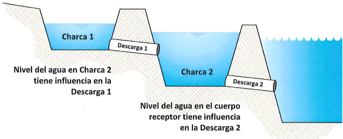
Figura 6.2 Esquemático de charcas interconectadas.
