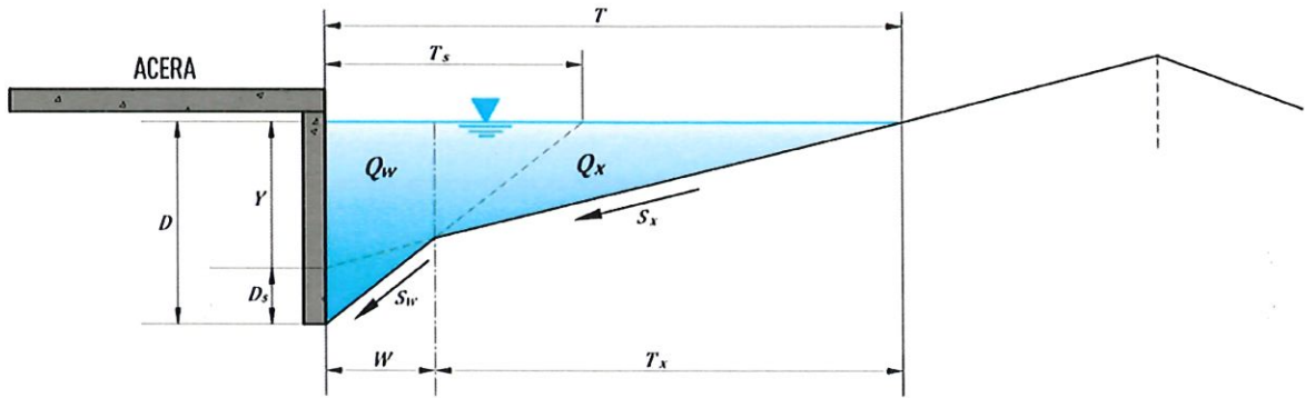
Figura 4.9 Detalle de sección de cuneta triangular compuesta.
