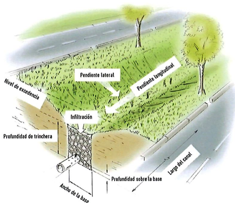
Figura 10.16 Esquemático de una zanja vegetada.
