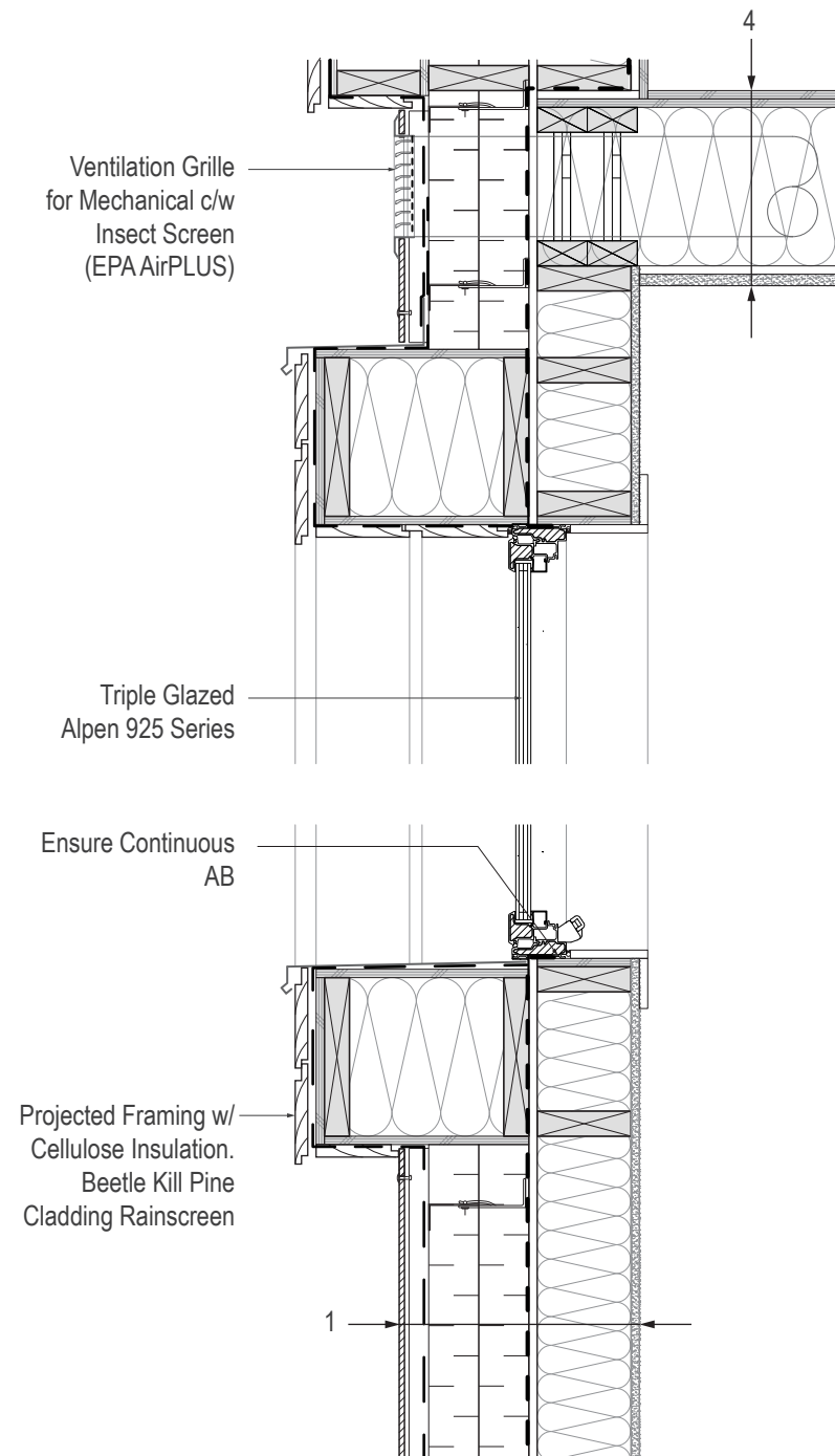
Detail 2 - North Aperture Sill & Top Plate Scale: 1" = 1'-0"
