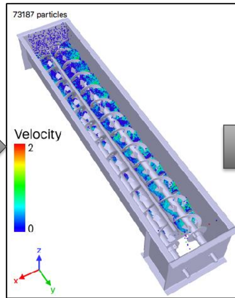
(b) Filling
